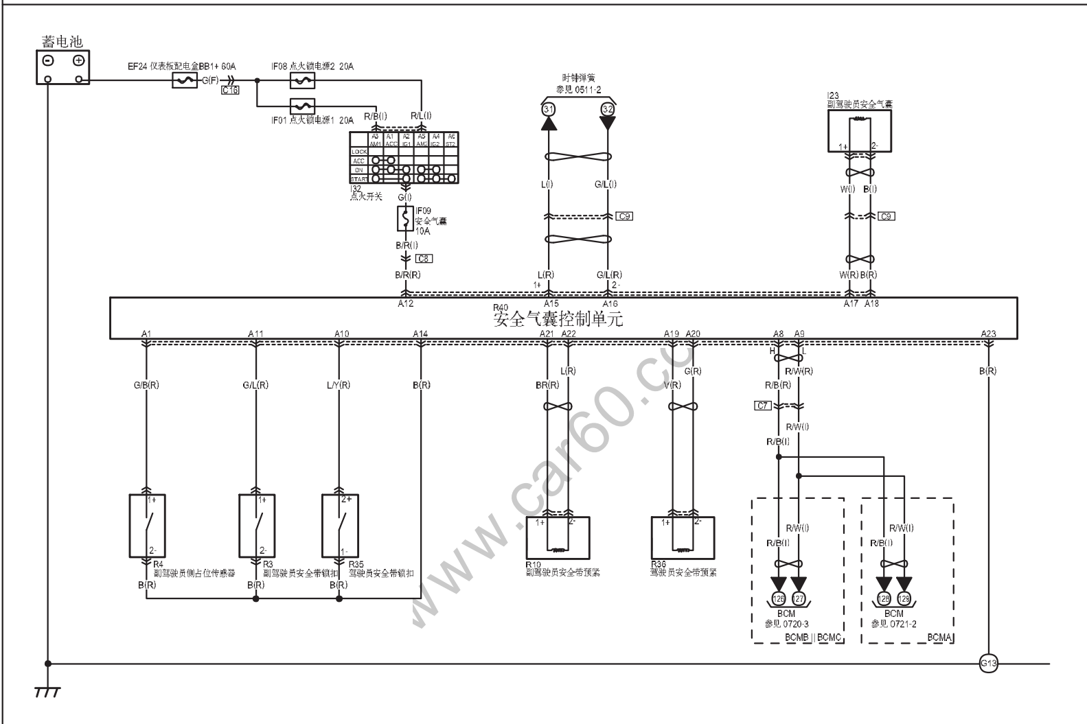
安全气囊控制单元
